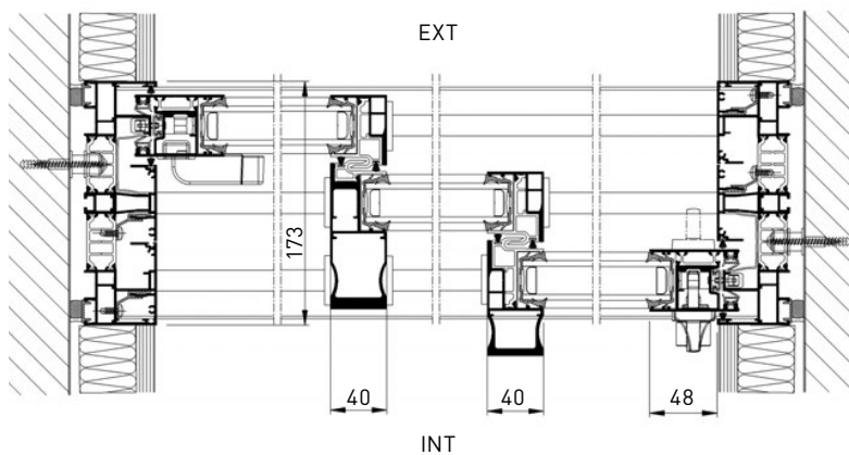
3 HOJAS / 3 RAÍLES - SECCIÓN HORIZONTAL
