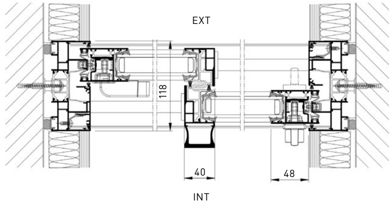
2 HOJAS MÓVILES - DETALLE INFERIOR
