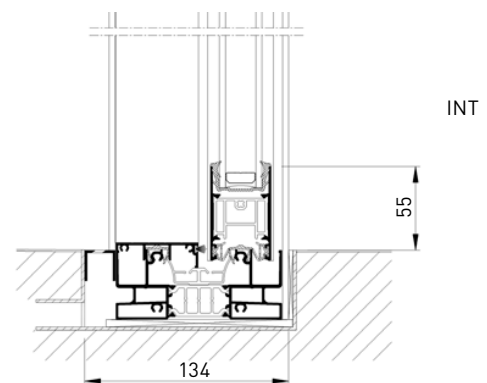
1 HOJA MÓVIL Y 1 FIJA - DETALLE INFERIOR
