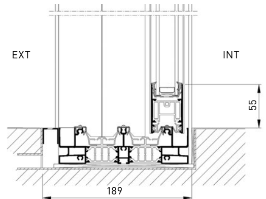
3 HOJAS MÓVILES - DETALLE INFERIOR
