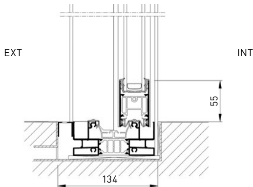
2 HOJAS MÓVILES - DETALLE INFERIOR
